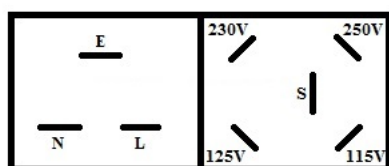
Mains I/P Module
